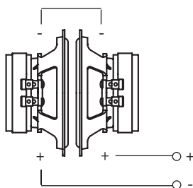
2B Collegamento Push-Pull serie mono 8 Ω (16)
