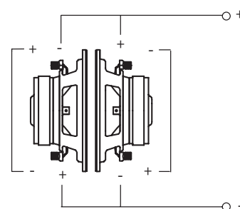
4C Collegamento Push-Pull serie/parallelo Mono 4 Ω (8)
