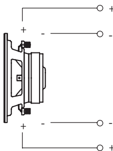
3C Collegamento Stereo 4+4 Ω (8+8)
