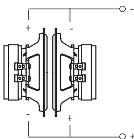
2C Collegamento Push-Pull parallelo mono 2 Ω (4)
