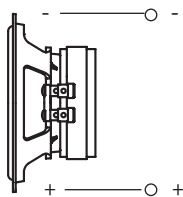
2A Collegamento Push-Pull stereo 4+4 Ω (8+8)
