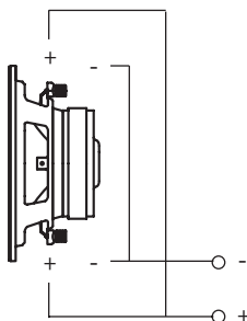
3A Collegamento Mono 2 Ω (4)
