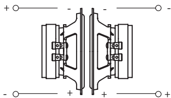
2B Collegamento Push-Pull serie mono 8 Ω (16)
