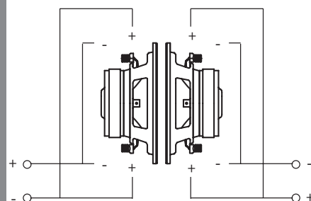
4A Collegamento Push-Pull parallelo Stereo 2+2 Ω (4+4)
