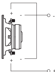
3B Collegamento Mono 8 Ω (16)
