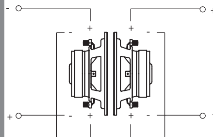
4C Collegamento Push-Pull serie/parallelo Mono 4 Ω (8)
